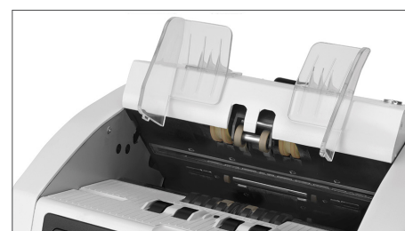
Interne onderdelen en sensoren kunnen eenvoudig worden gereinigd door het boven- en achterpaneel te openen
