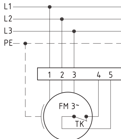
Anschlußplan 0.13-2 I.
