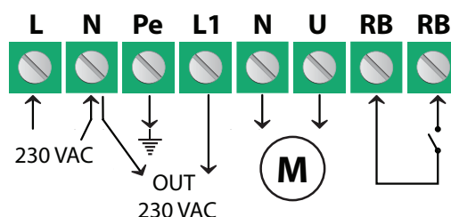
Fig. 3 Aansluitschema
