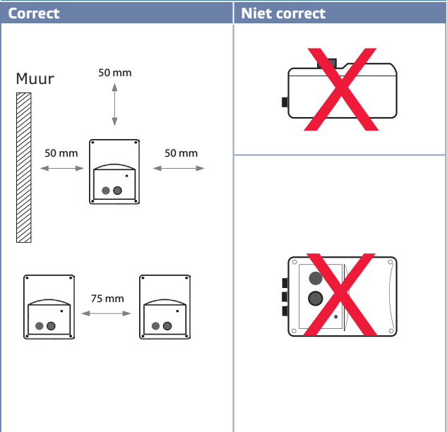
Fig. 2 Montagepositie
